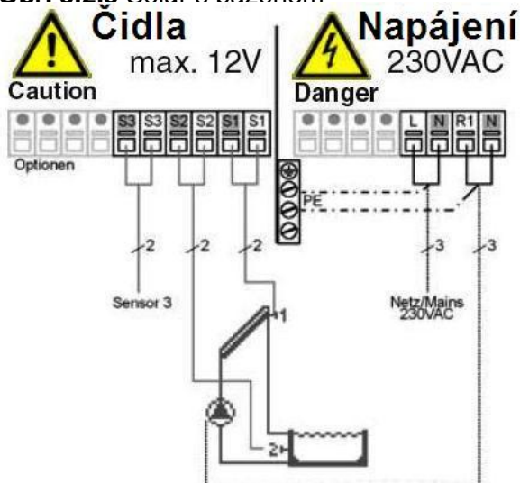
Obr. 3.2.3 Solár s bazénem
