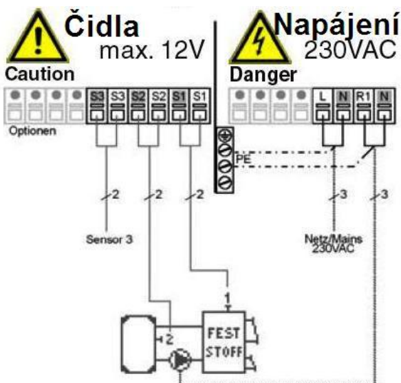
Obr. 3.2.4 Kotel na pevná paliva a zás. ohřivač
