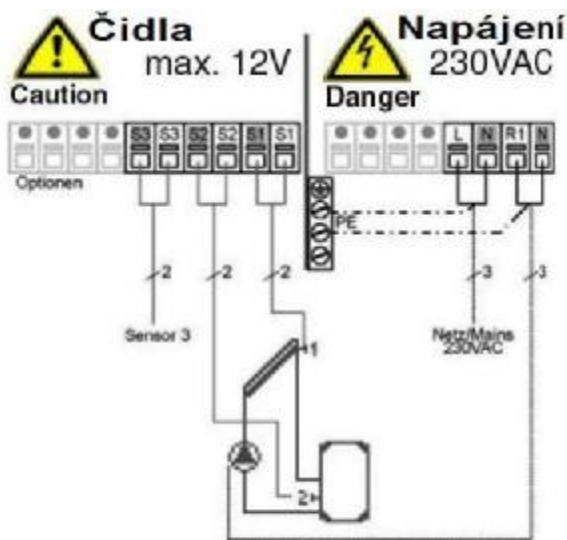
Obr. 3.2.2 Solár se zásobníkovým ohřívačem
