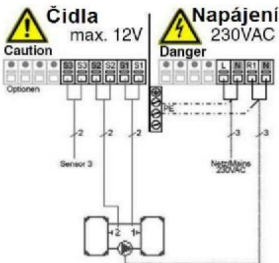
Obr. 3.2.6 Předávání mezi zásobníky
